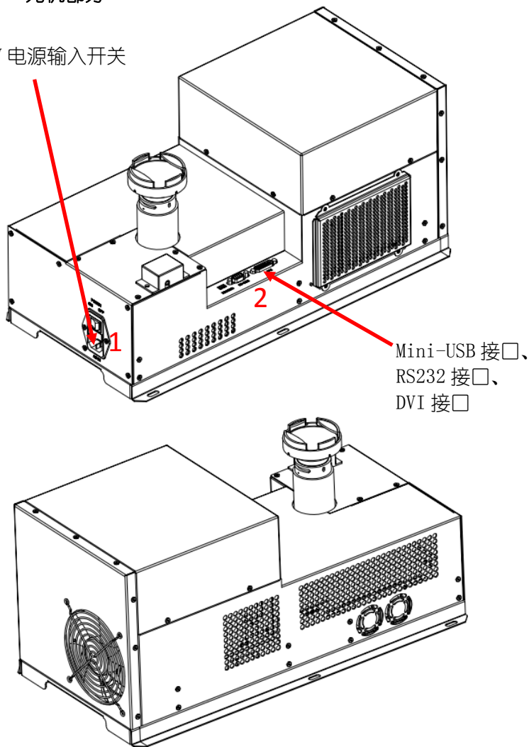
图 4 光机连线图
